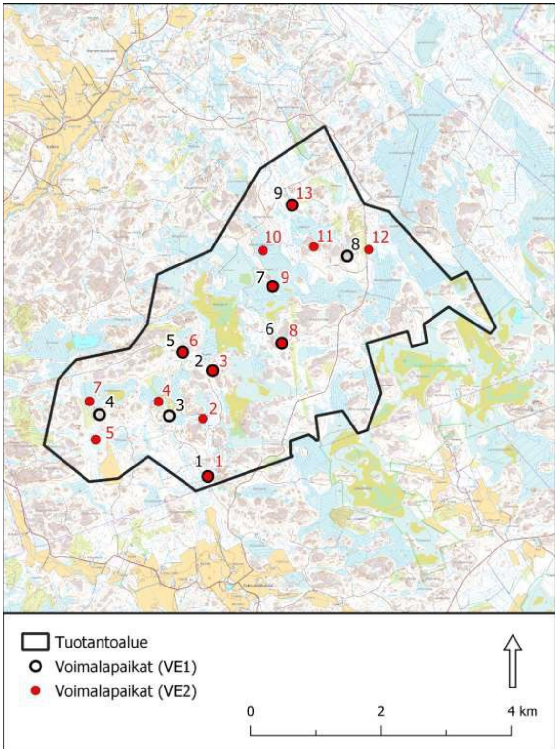
Kuva 4-2. Alustava voimalasijoittelu tuotantoalueella. VE1-vaihtoehdossa maksimivoimamäärä olisi 9 voimalaa (mustat merkinnät) ja VE2:ssa 13 voimalaa (punaiset merkinnät). Taustakartta © MML 2024.
